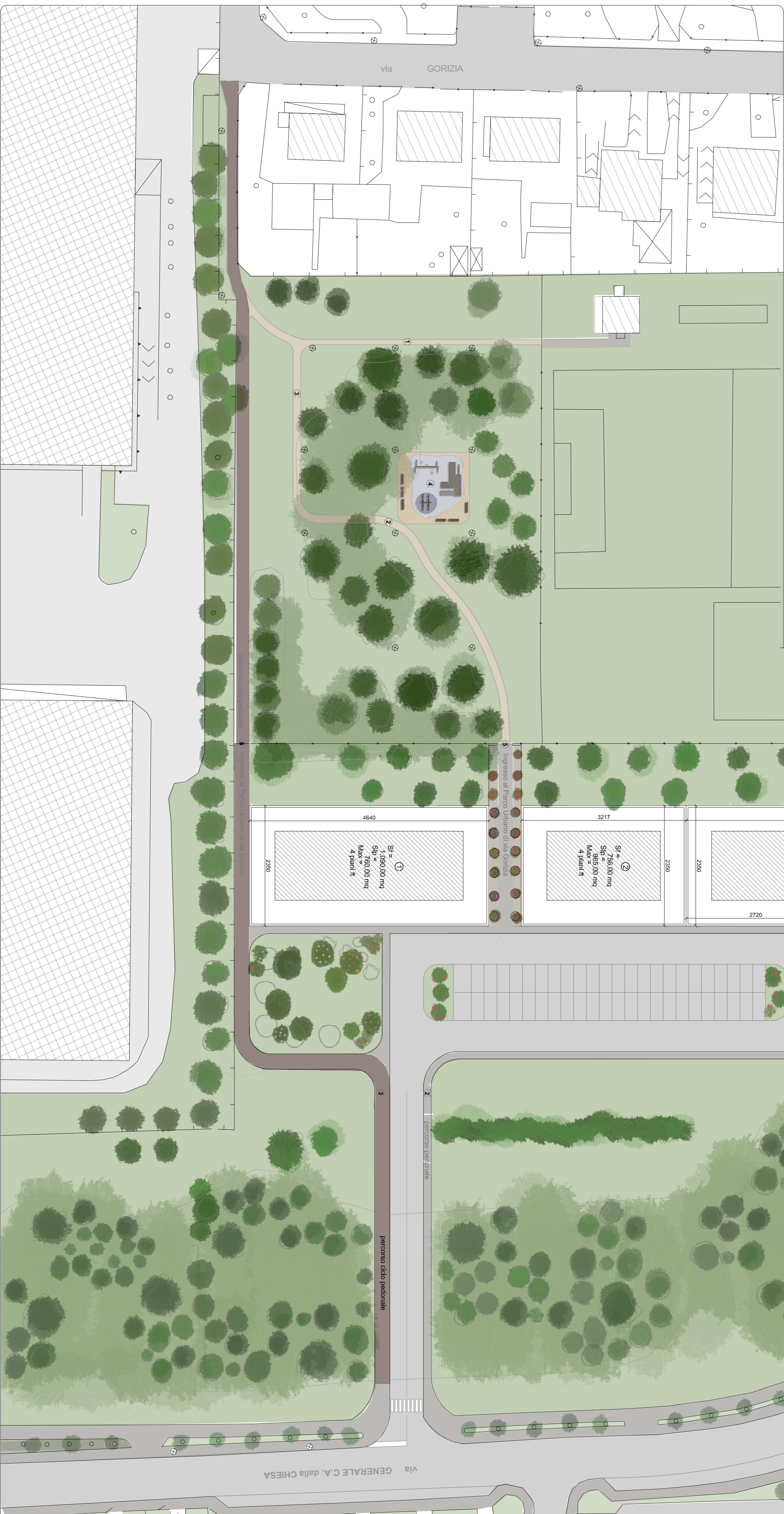
Planivolumetrico area di intervento, via Generale della Chiesa e riqualificazione Parco Urbano di via Gortiza | scala 1:500
