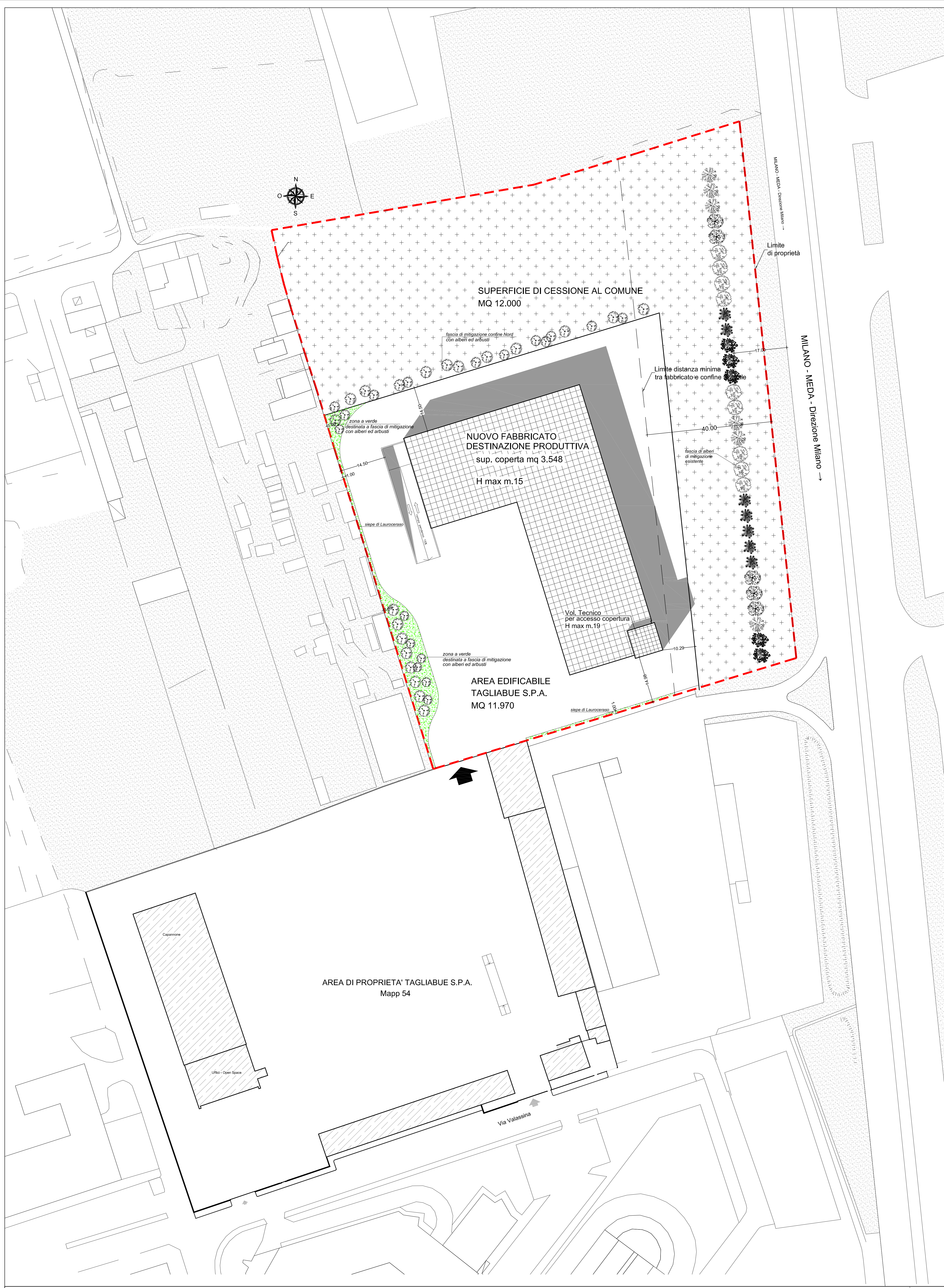
PLANIVOLUMETRICO DI PROGETTO scala 1:500
